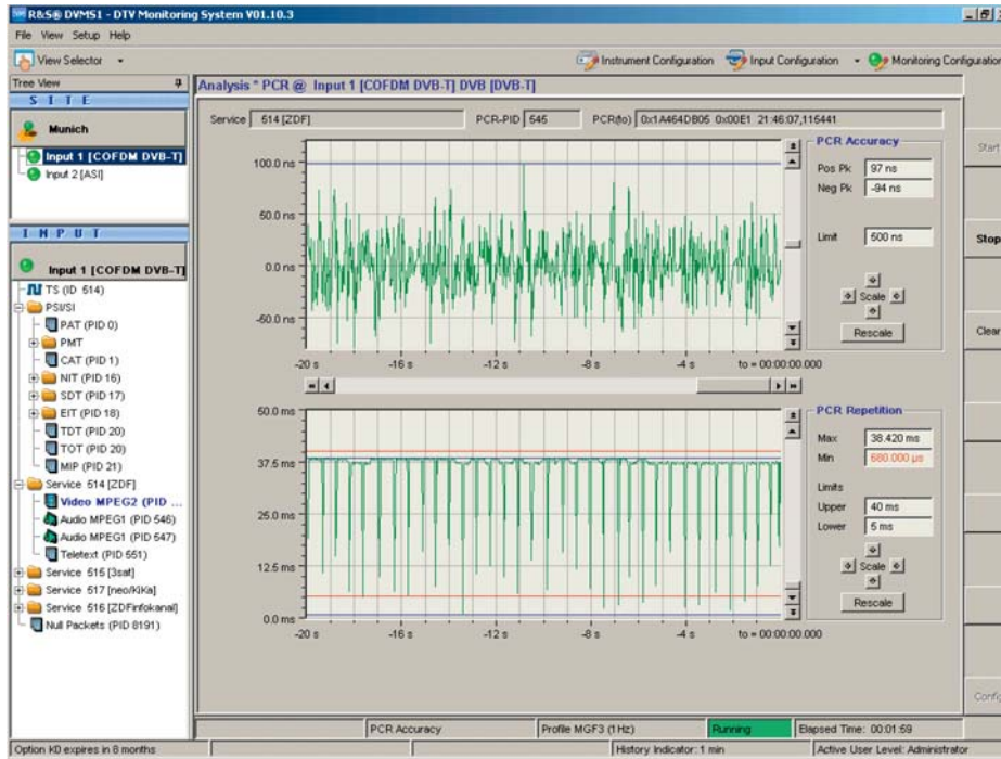
Графический интерфейс пользователя, показывающий результаты анализа PCR
